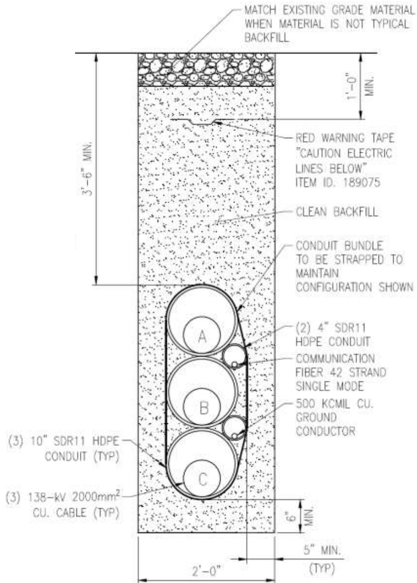
(d) Direct-Buried Conduits in Vertical Configuration
